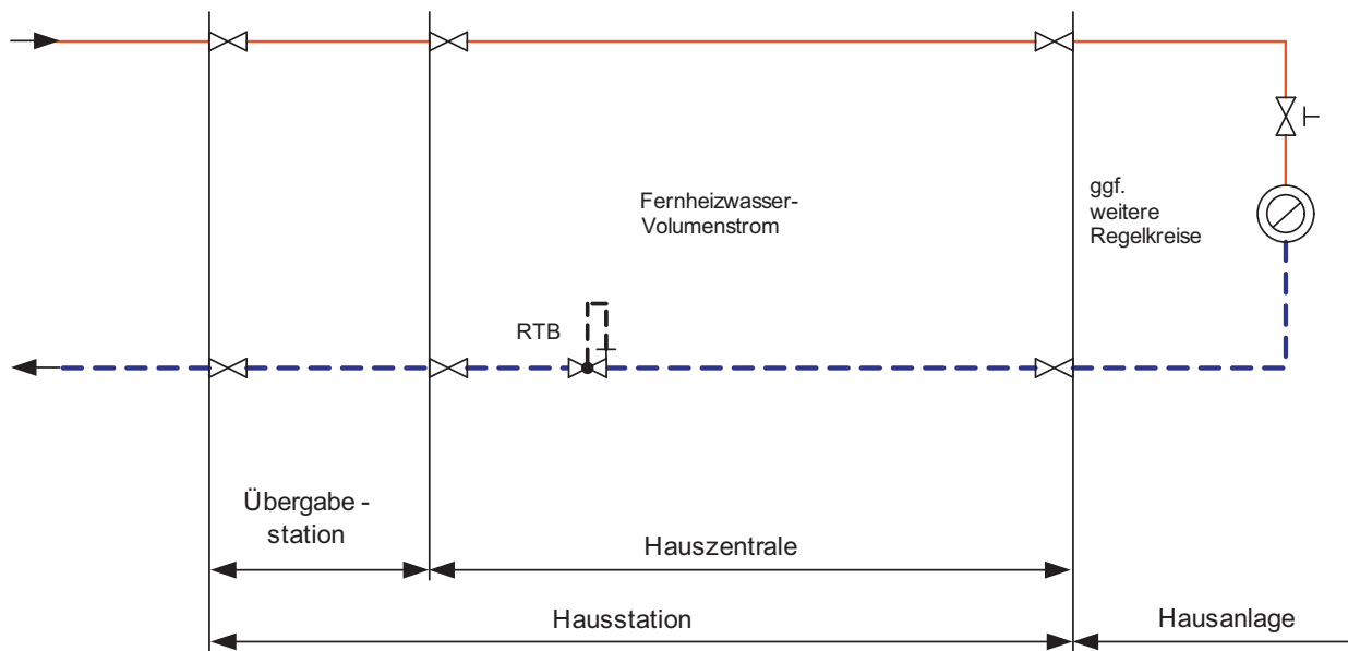
Abbildung 8: Hauszentrale-Raumheizung, Prinzipialschaltbild für den direkten Anschluss ohne Beimischregelung gilt nur für Garath
