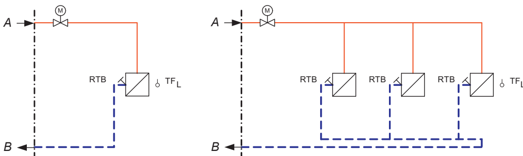
Abbildung 7: Hauszentrale-Raumluftheizung Prinzipaltbilder für den indirekten Anschluss
