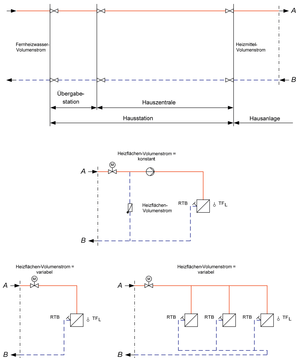
Abbildung 11: Hauszentrale-Raumluftheizung mit drei beispielhaften Hausanlagen, Prinzipschaltbilder für den direkten Anschluss ohne Beimischregelung
